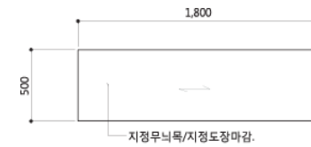
가족실테이블 TOP VIEW
