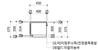
가족실선반장 SIDE VIEW
