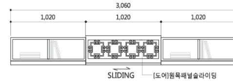
2 가족실선반장 FRONT VIEW
